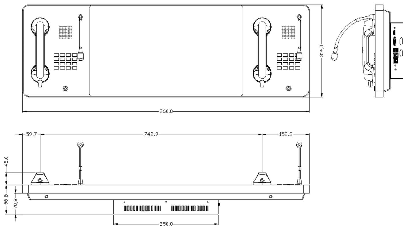
安装尺寸图:
